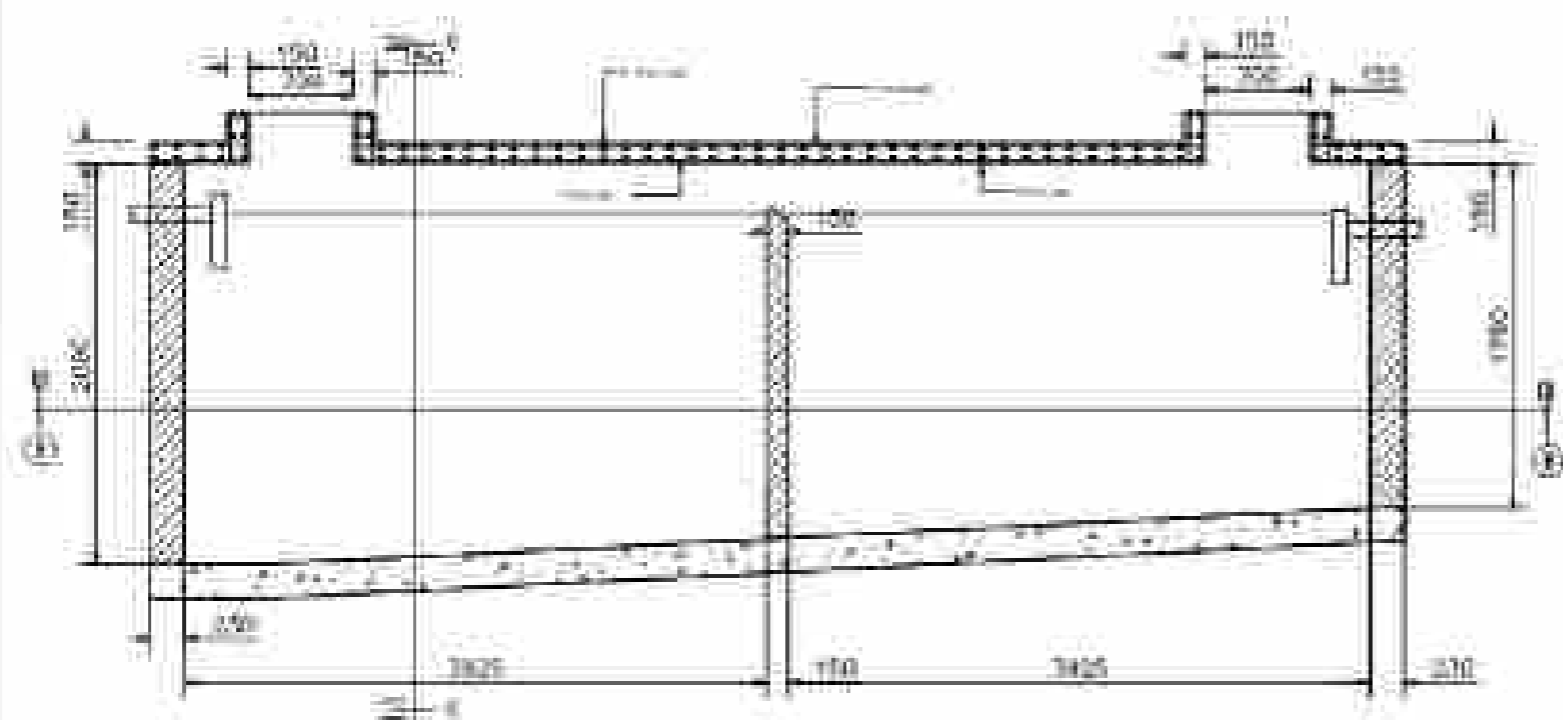
SECTION A-A 1:100
